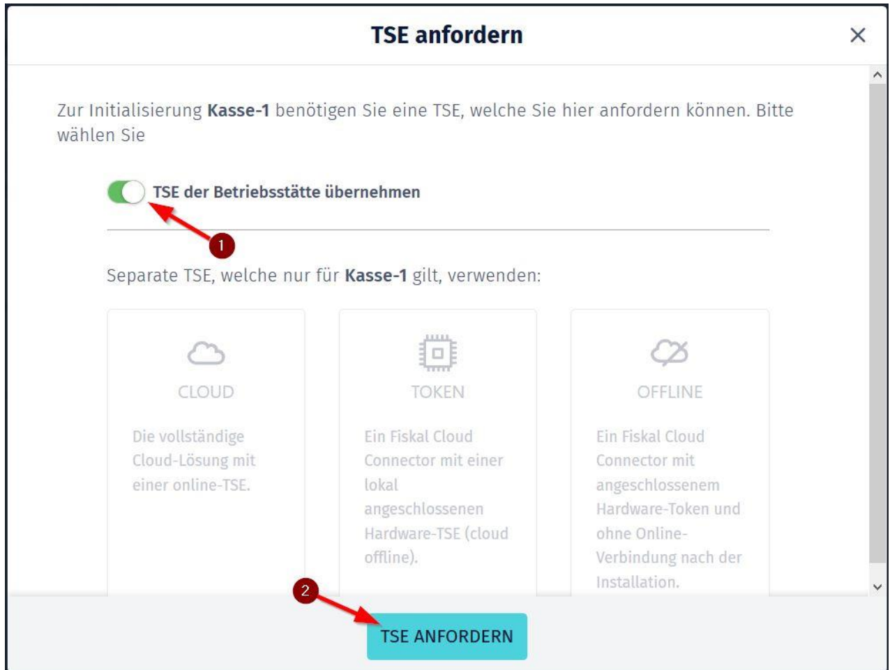
Abbildung 5: TSE anfordern
